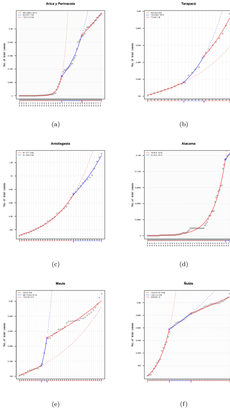
FIGURA 4. Regresión segmentada y puntos de cambio para regiones de Arica a Atacama, el Maule y Ñuble.
